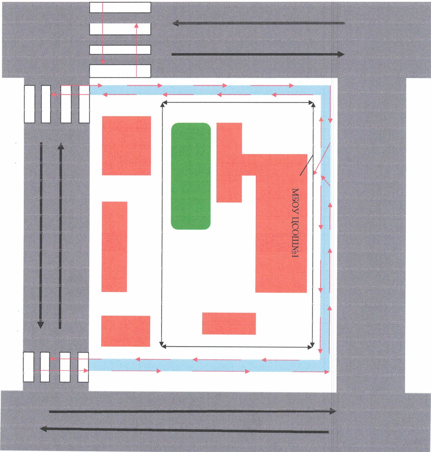
2 Схема организации дорожного движения в непосредственной близости от образовательного учреждения с размещением соответствующих технических средств, маршруты движения детей и расположение парковочных мест
